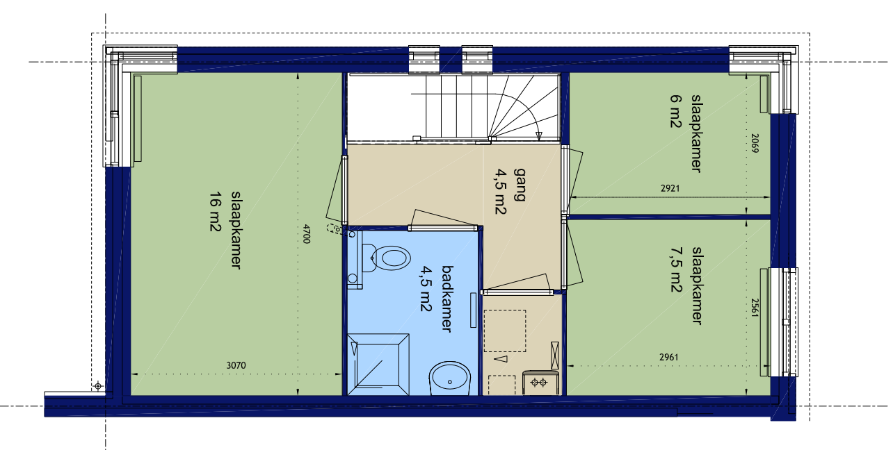
type B1 - 1e verdieping Van Reenenweg
