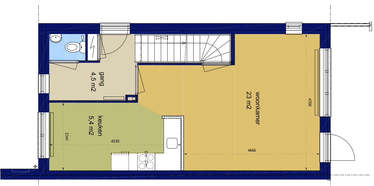
type B1 - begane grond Van Reenenweg
