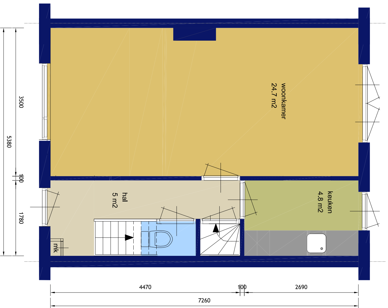
begane grond
