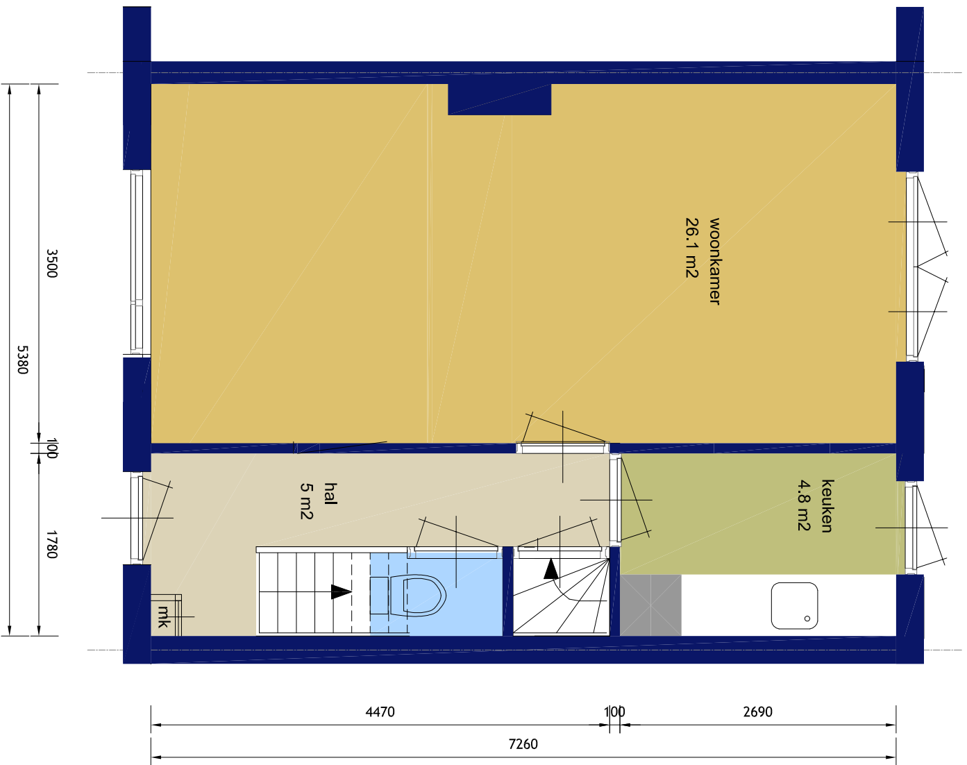
begane grond
