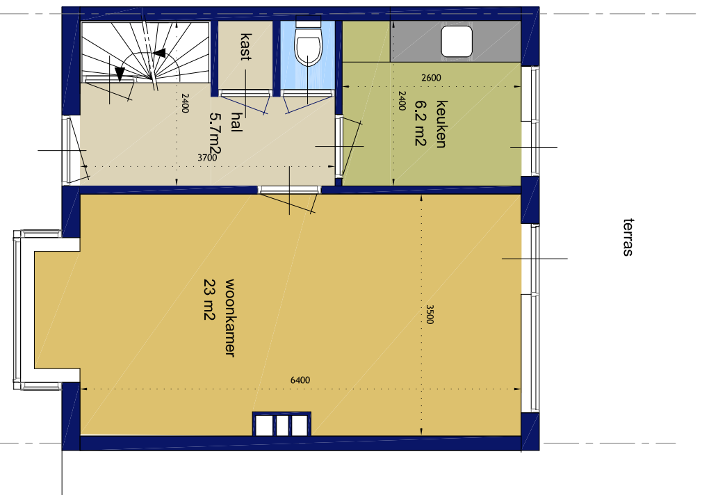
woningtype Lc begane grond
