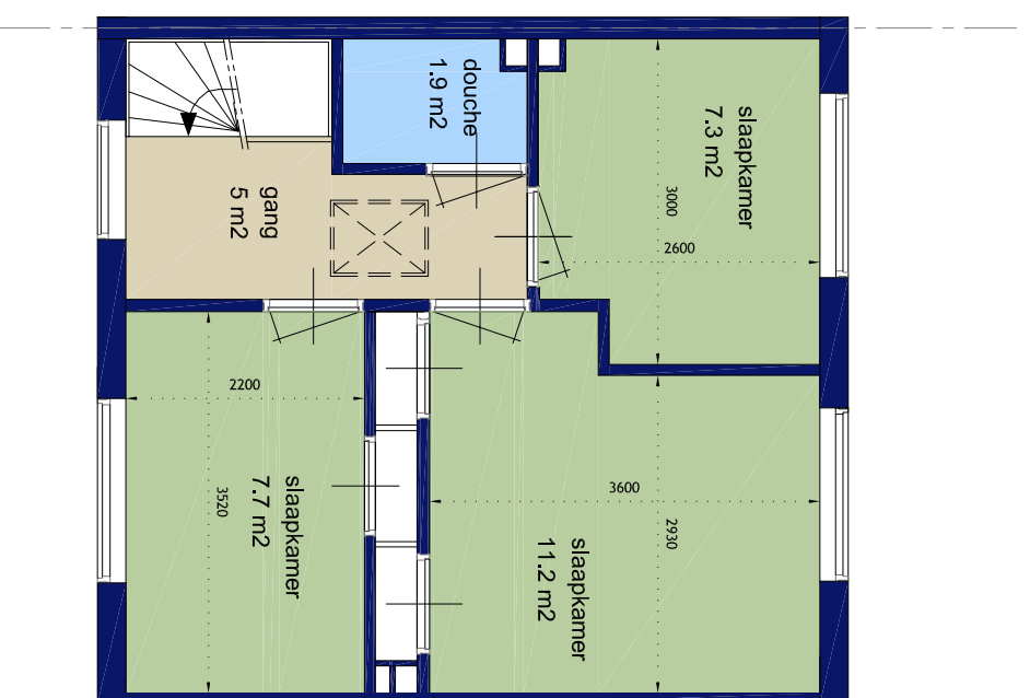
woningtype Lc 1e verdieping
