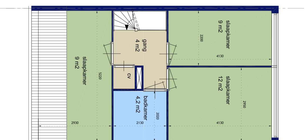
type B - 2e bouwlaag De Clomp
