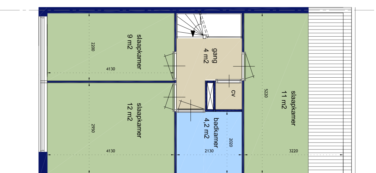
type E - 2e bouwlaag De Clomp
