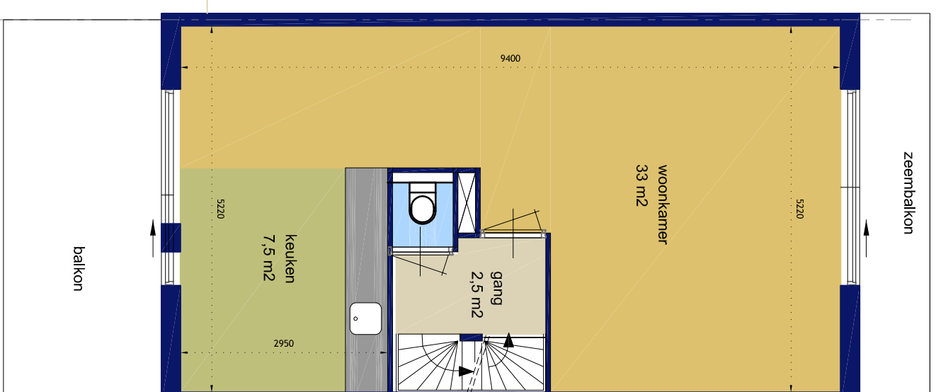
type L(s) - 1e verdieping De Clomp
